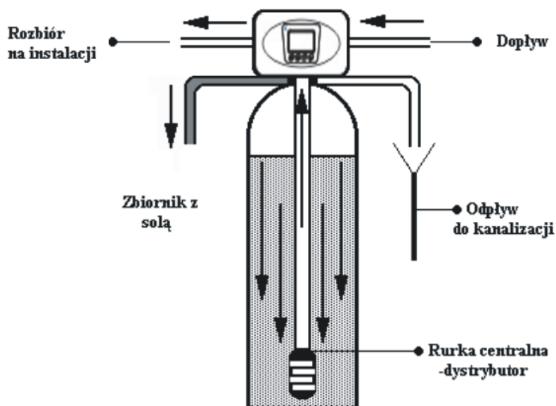
Rys. L. Przepływ wody przez urządzenie w cyklu napełniania zbiornika z solanką.
