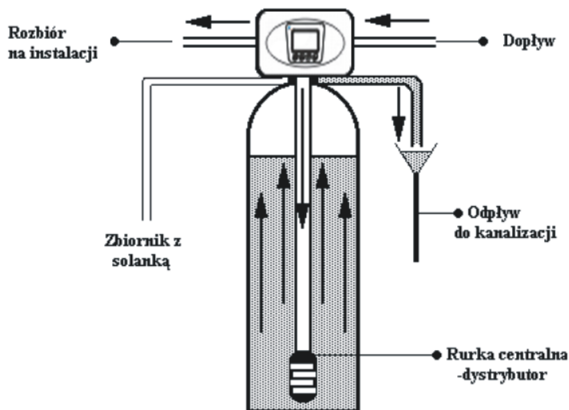
Rys. J. Przepływ wody przez urządzenie w cyklu płukania wstecznego.
