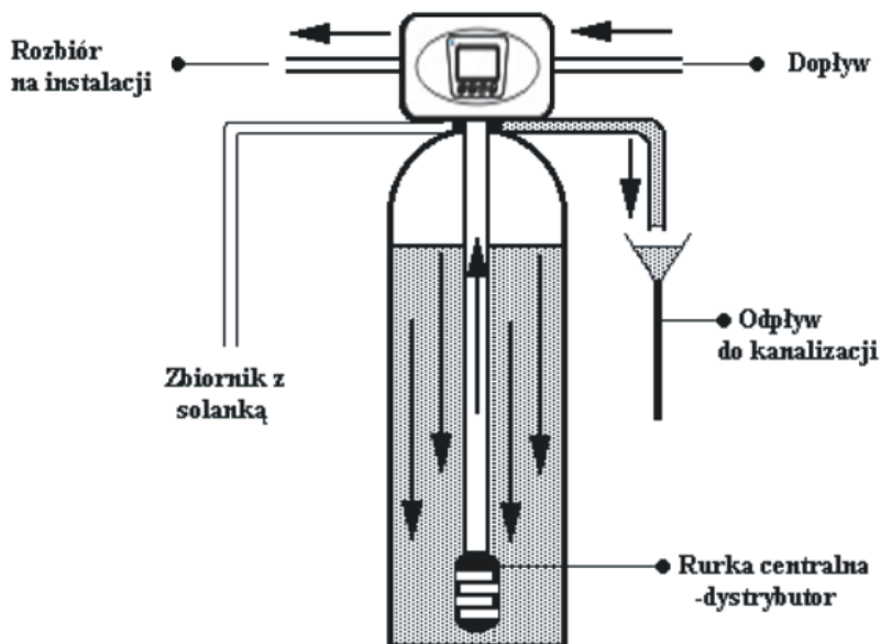
Rys. M. Przepływ wody przez urządzenie w cyklu szybkiego płukania złoża.
