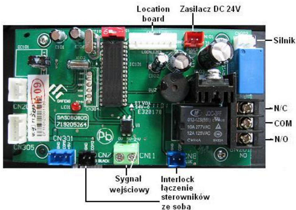
Rys. H. Podłączenie wejściowego i wyjściowego zewnętrznego sygnału elektrycznego.
