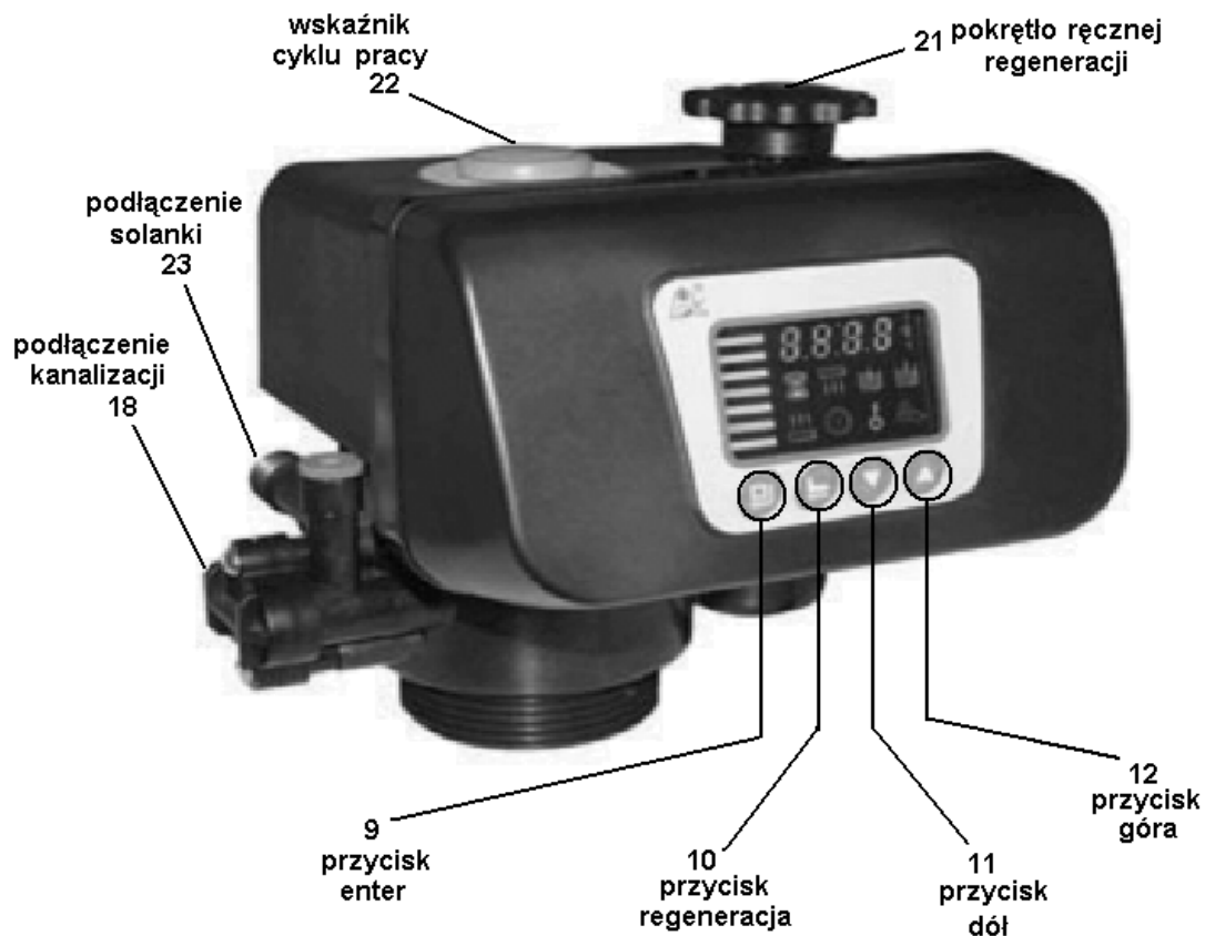
Rys. A. Sterownik RX63B
